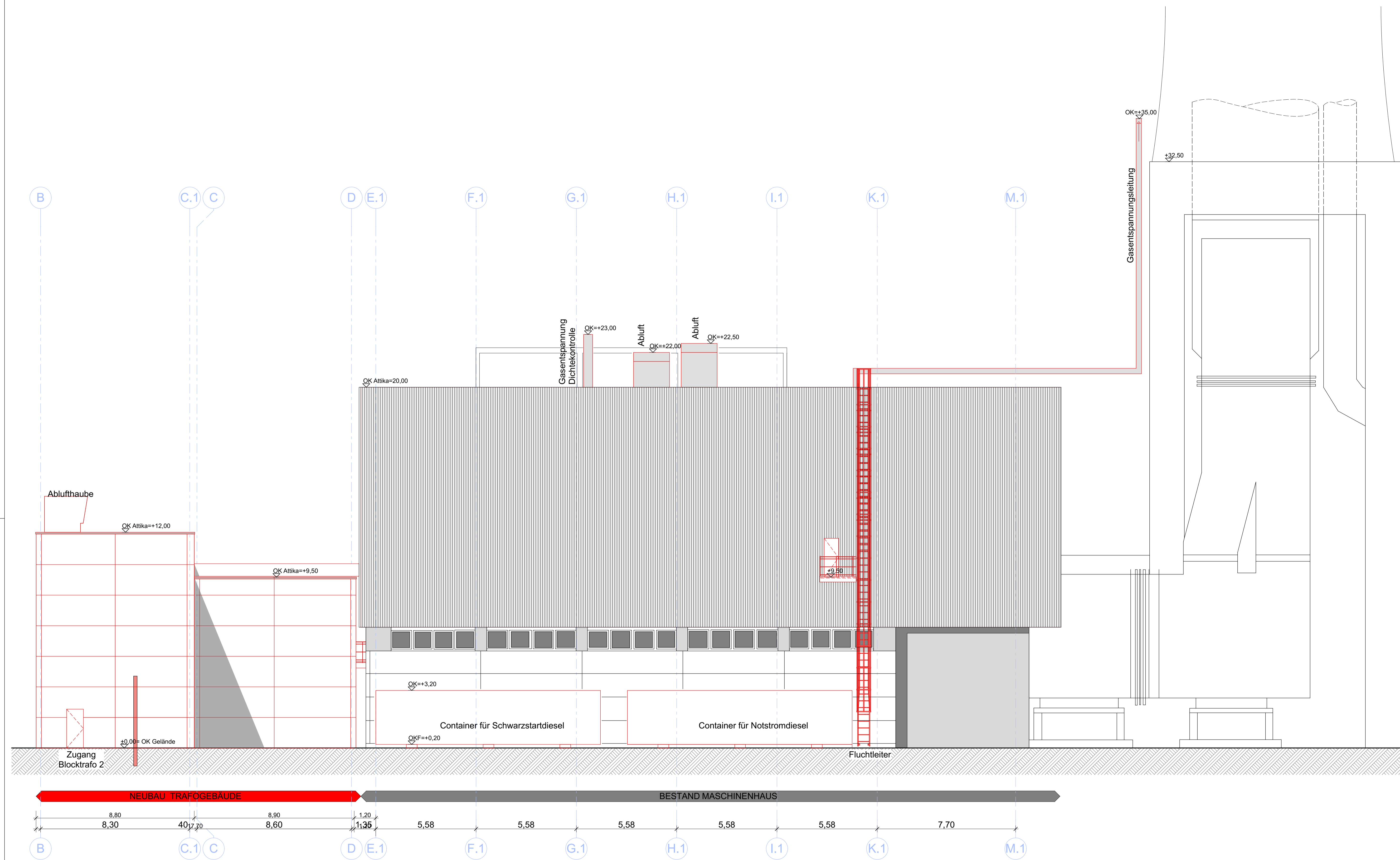
Ansicht Ost Maschinenhaus + Trafogebäude 2
