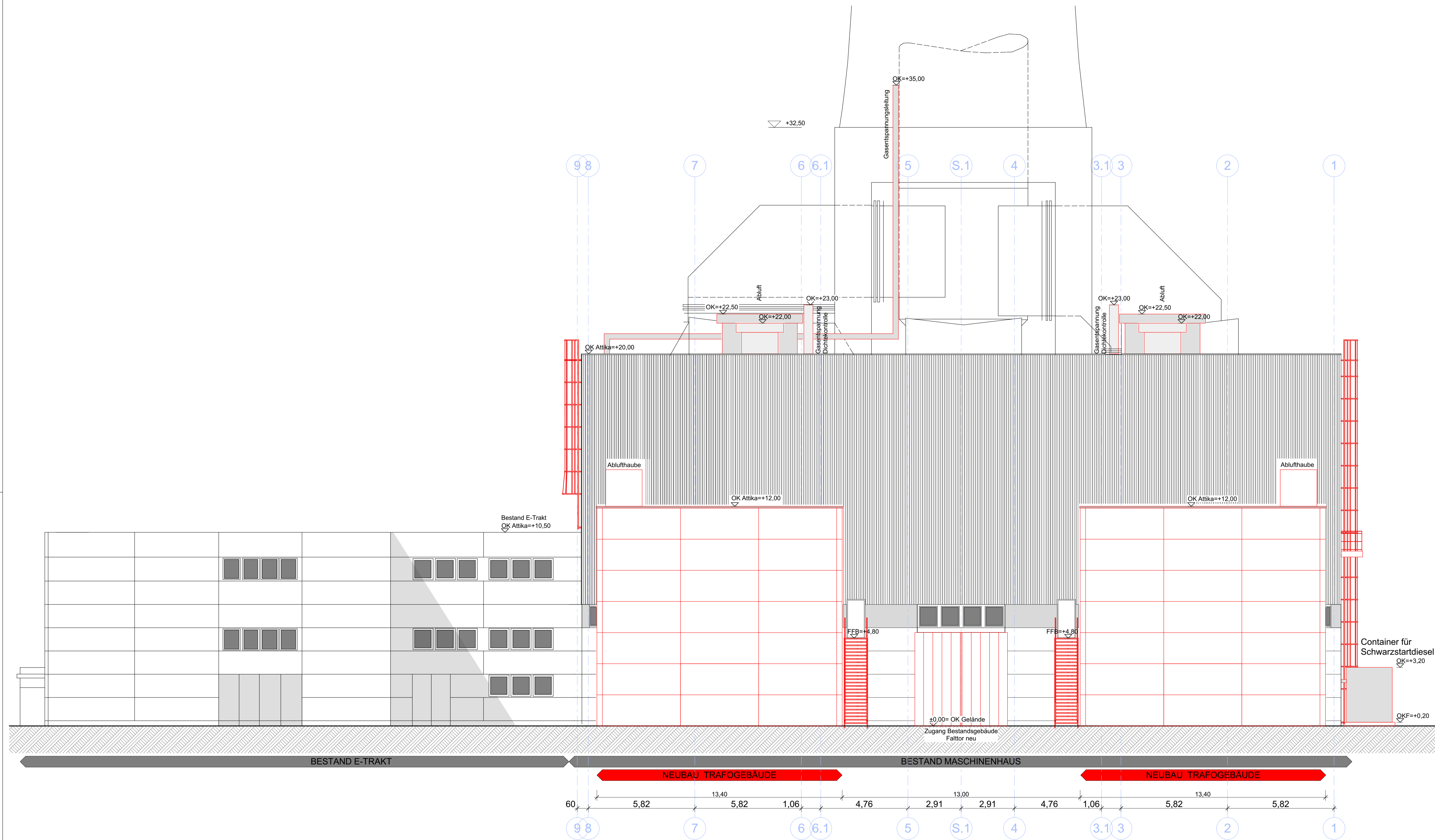
Ansicht Süd Maschinenhaus + Trafogebäude 1 + 2
