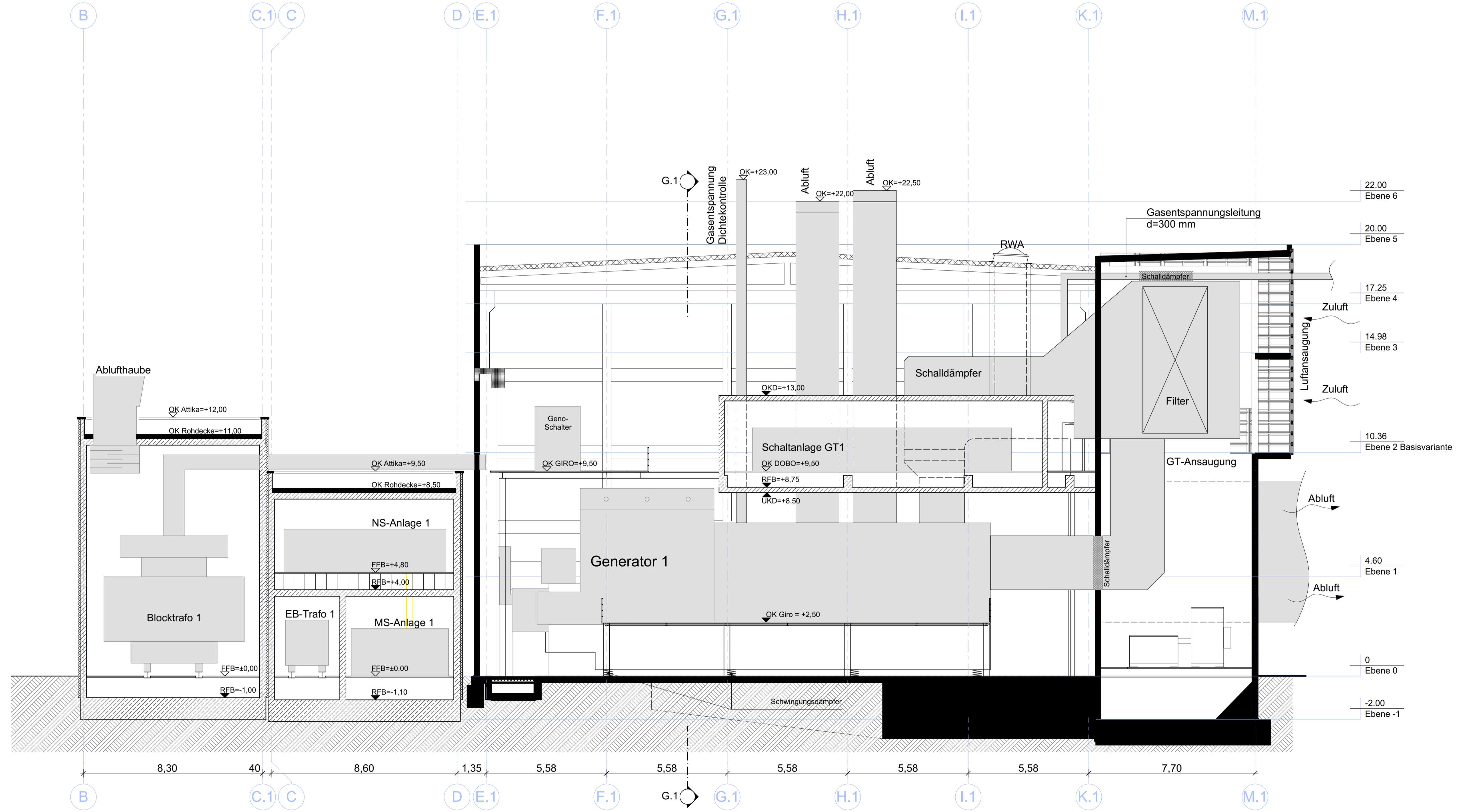
Schnitt Achse 6.1 - Maschinenhaus + Trafogebäude 1
