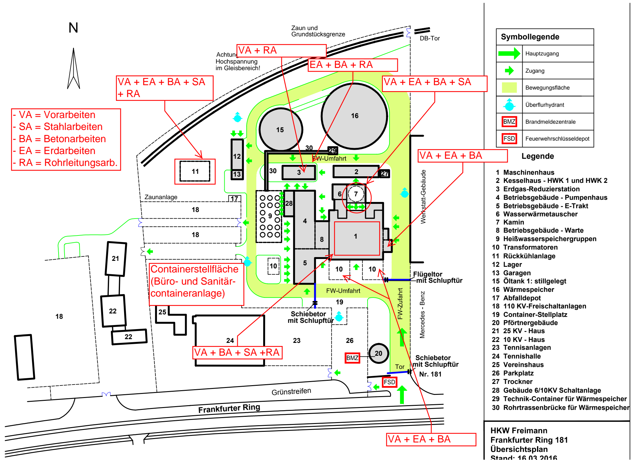
SWM Baustelleneinrichtungsplan mit Darstellung der Umbau- arbeiten an den Anlagen Stand: 24.06.2016
