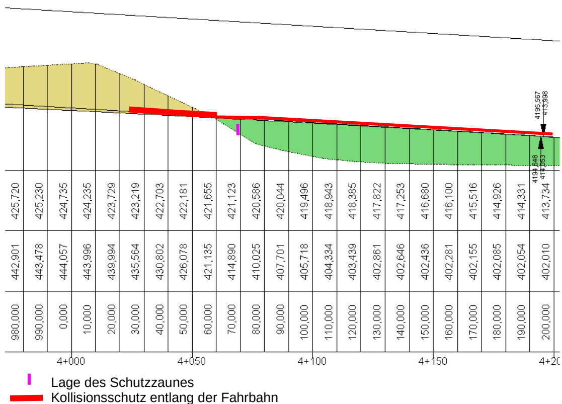
Abbildung 2: Höhenplan mit Vermeidungsmaßnahmen
