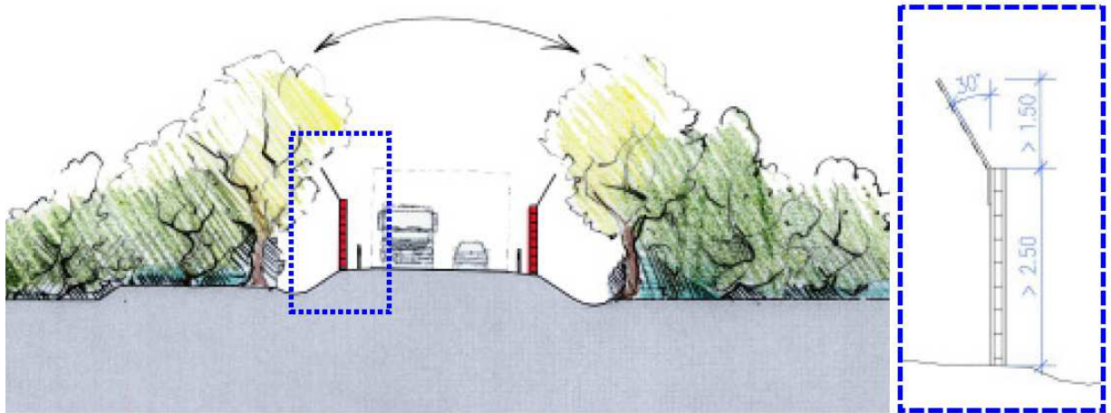
Abbildung 3: Beispielhafte Gestaltung der Kollisionsschutzeinrichtung
