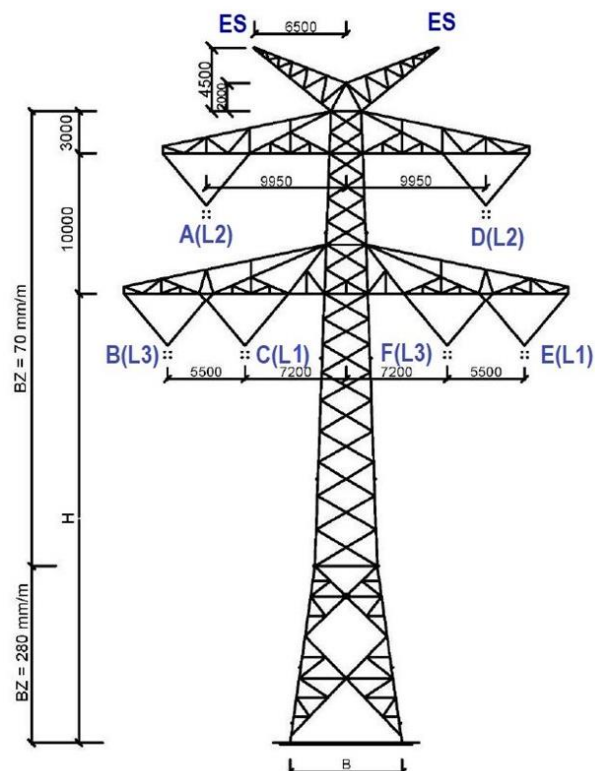
Abbildung 4: Mastgestänge Donau D-2-D-2018.3 - Grundtyp T2
