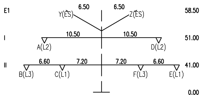
Abbildung 2: V-Kette mit Kettenlänge 4,5m
