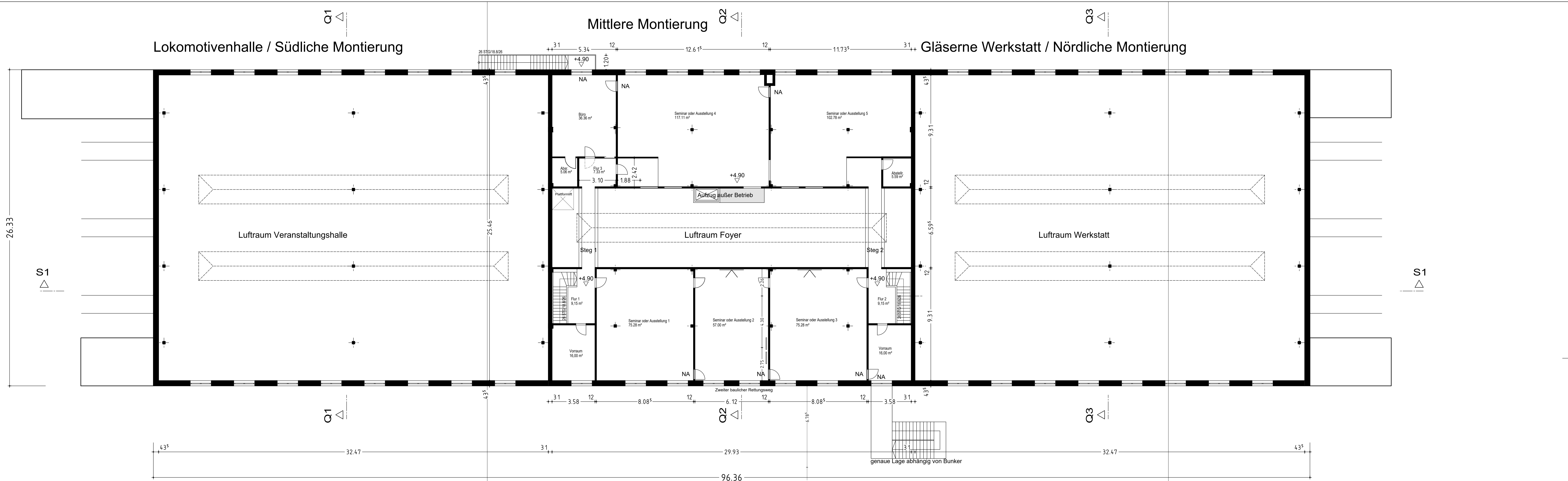
Dampflokhalle Grundriss Obergeschoss
