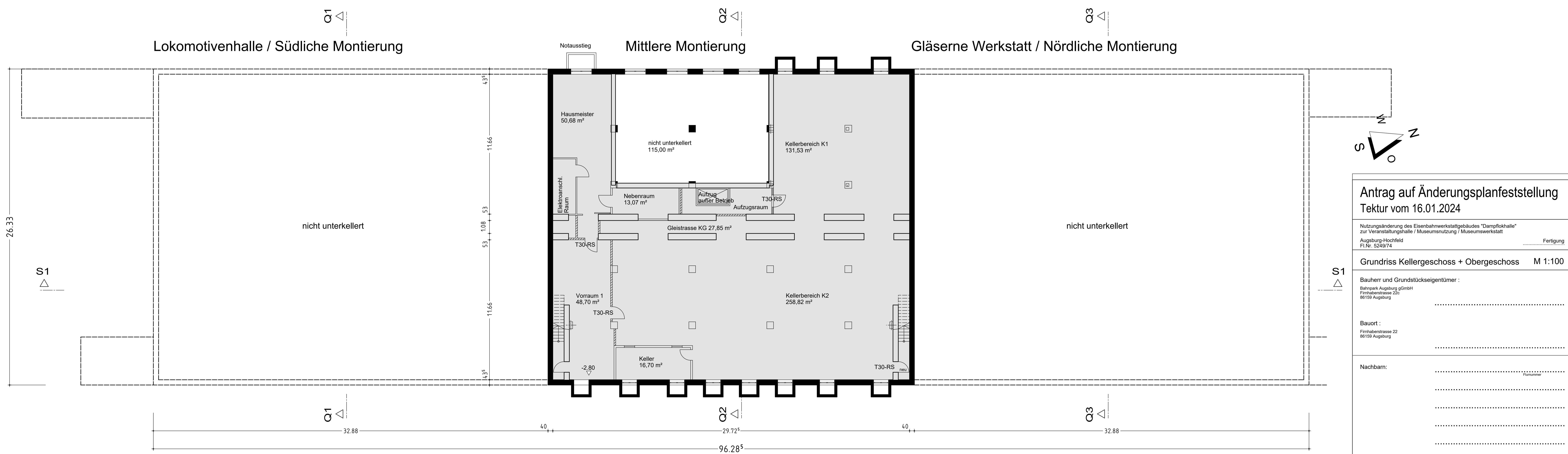
Dampflokhalle Grundriss Kellergeschoss
