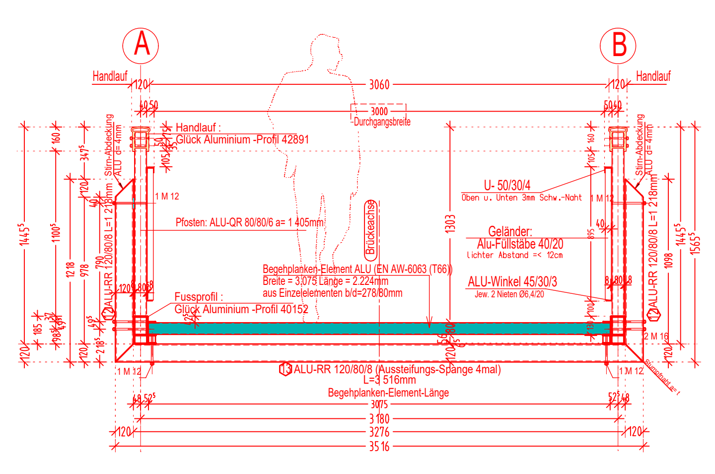
Querschnitt M 1:25
