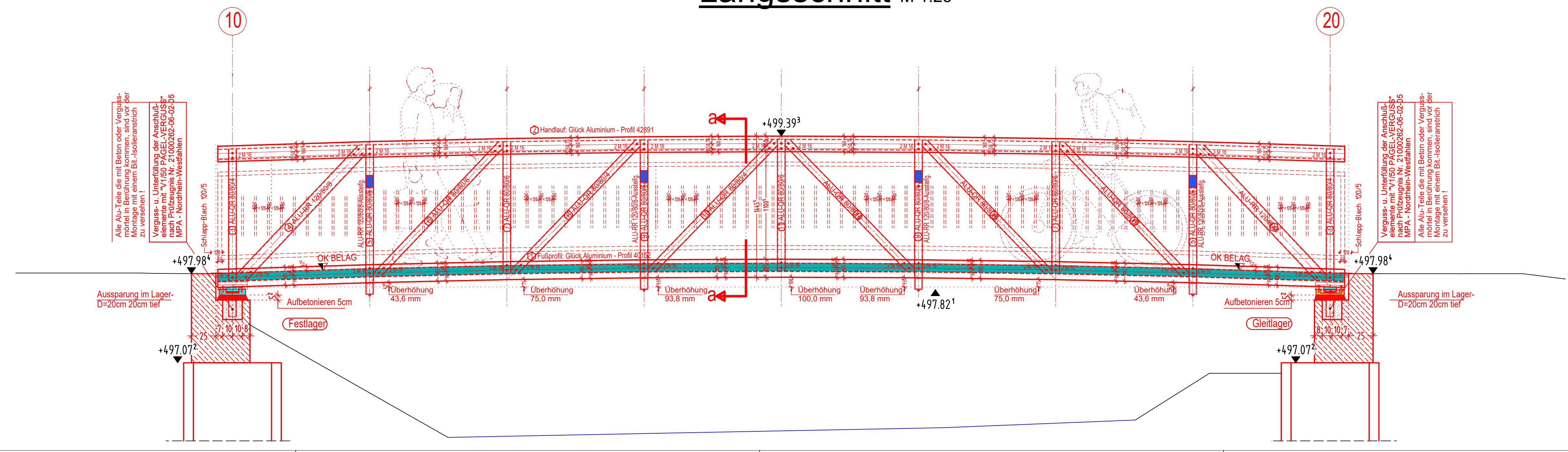
Längsschnitt M 1:25
