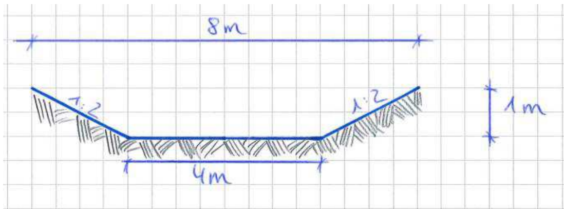
Abbildung 4-1: Skizze Graben
