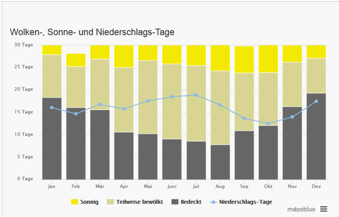
Diese Grafik zeigt die Anzahl der Tage mit Sonnenschein, teilweiser Bewölkung, Bedeckung und Niederschlag. Tage mit weniger als 20% Bewölkung werden als Sonnen-Tage eingestuft, Tage mit 20-80% Bewölkung als teilweise bewölkt und Tage mit mehr als 80% bedeckt.
